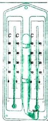
Hình 39.3 Ẩm kế khô – ướt
