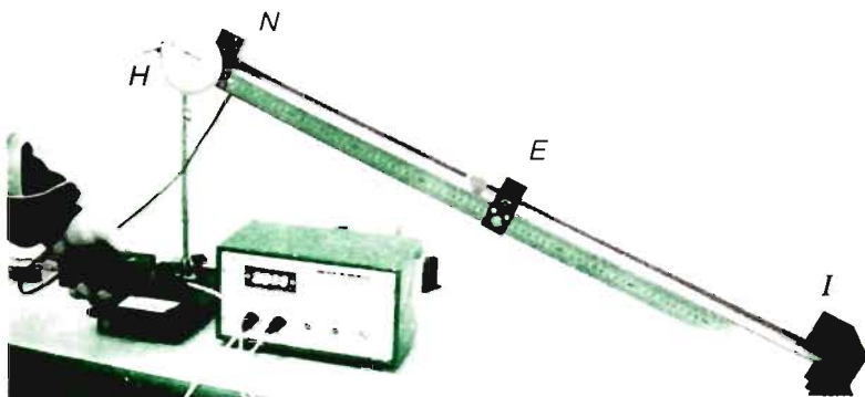
Hình 16.1 Bộ thí nghiệm xác định hệ số ma sát.
