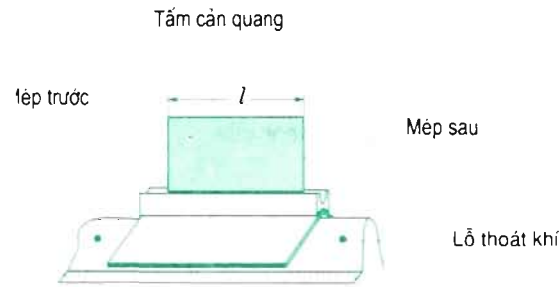
Hình 10.9. Vật trượt trên băng đệm khí.
