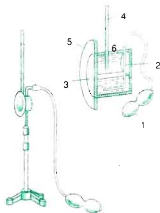
Hình 39.4 Ấm kế điểm sương
