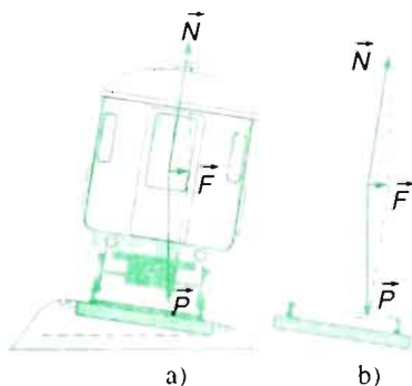
Hình 14.3 Đoạn đường sắt nghiêng.
