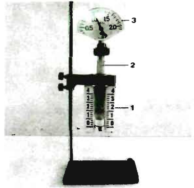
Hình 29.2. Sơ đồ thí nghiệm quá trình đẳng nhiệt.
