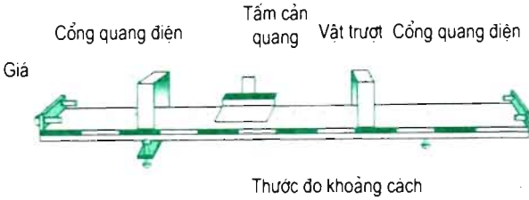
Hình 10.7. Hệ thống băng đệm khí
