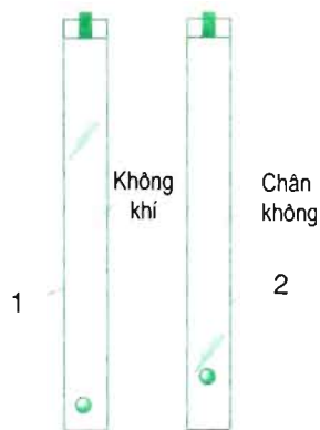
Hình 4.1. Ống Niu-tơn
